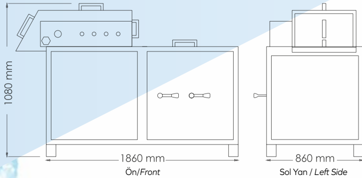
Genel Ölçüler / General Dimensions
